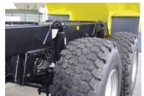
Tandem à suspension hydraulique (stabilité au bennage).
